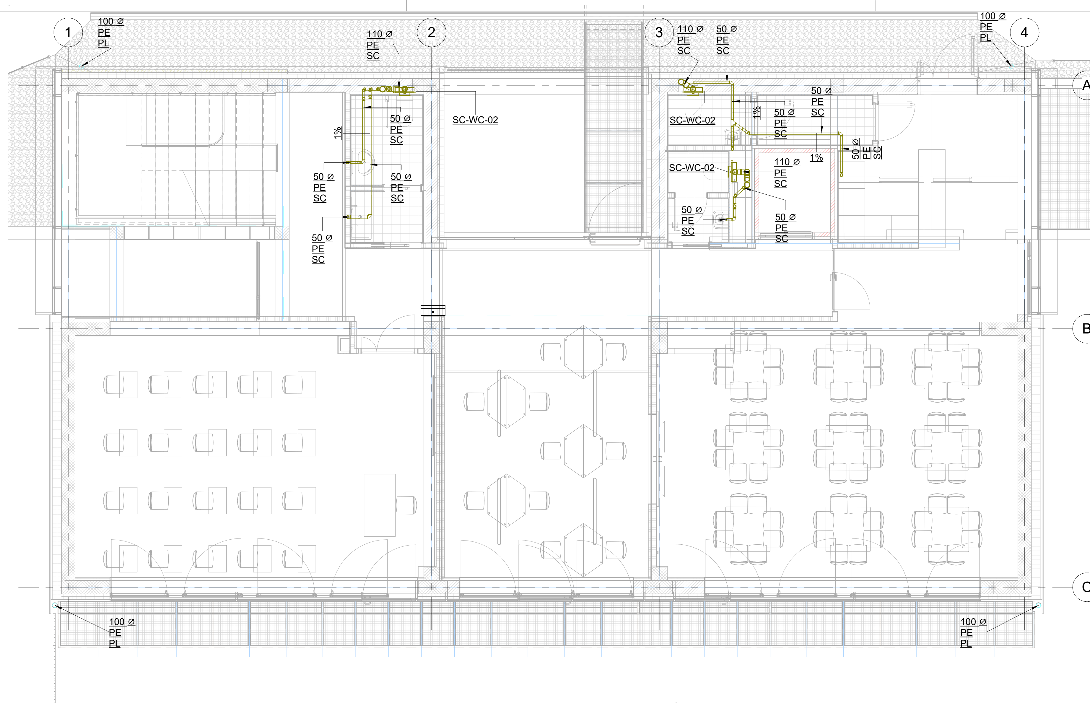
1 Pianta - Scarichi - Piano Primo 1 : 50
