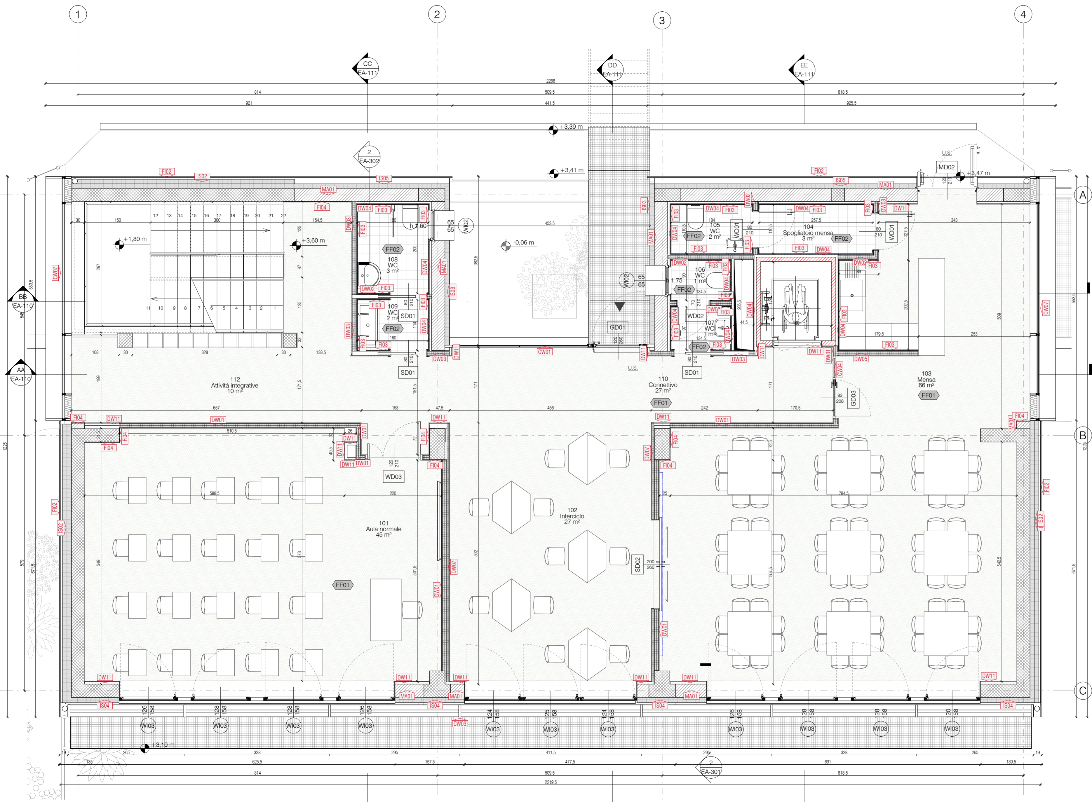
Pianta- Piano Primo 1 : 50
