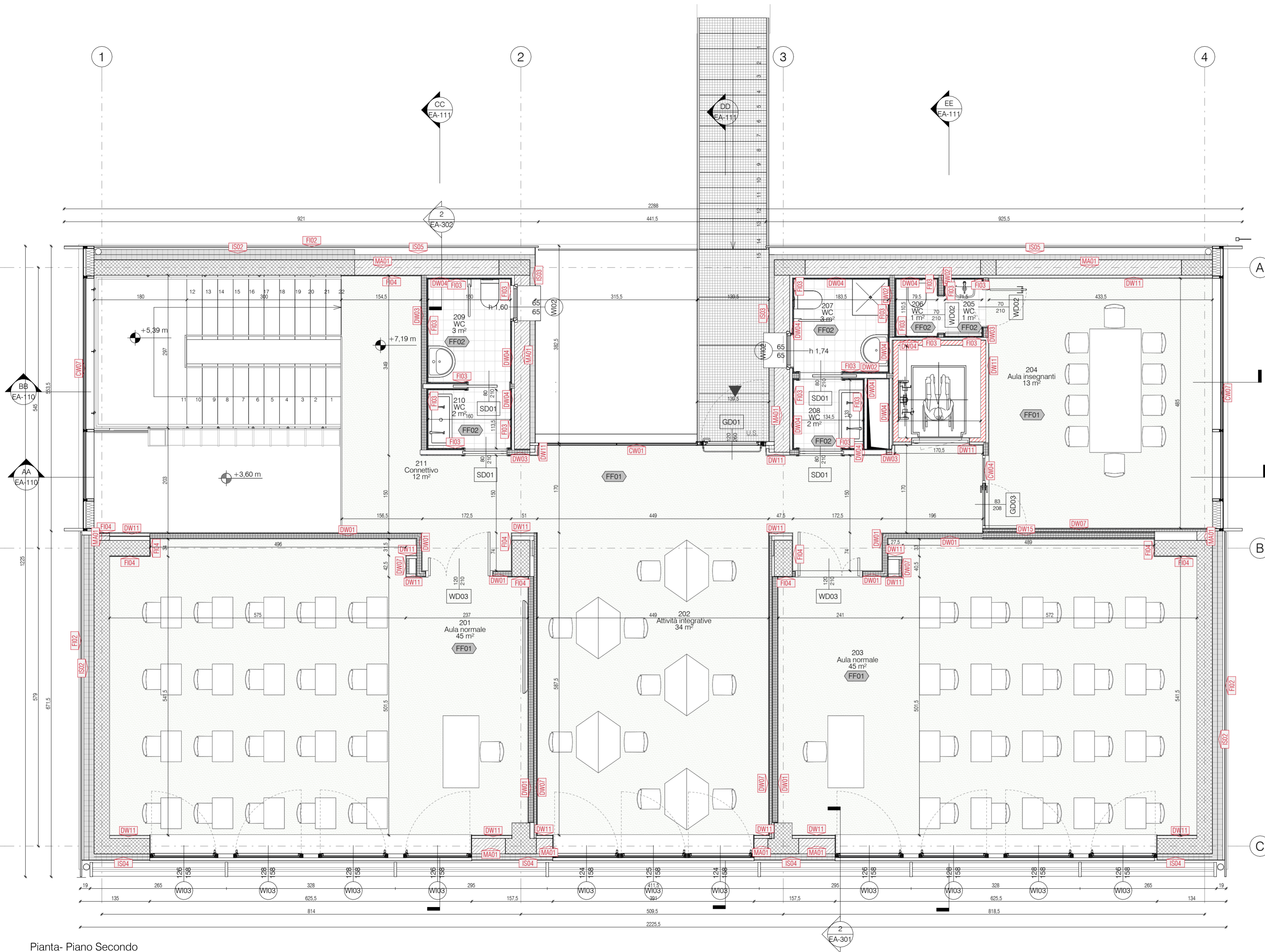
Pianta- Piano Secondo 1 : 50
