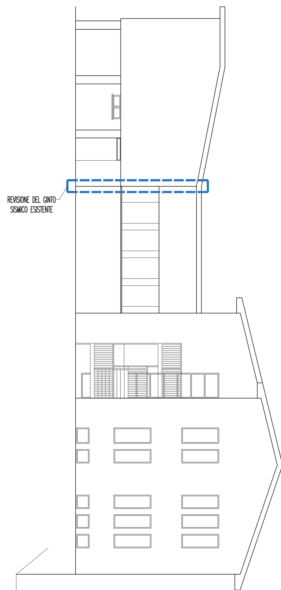
Prospetto OVEST Scala 1:100
