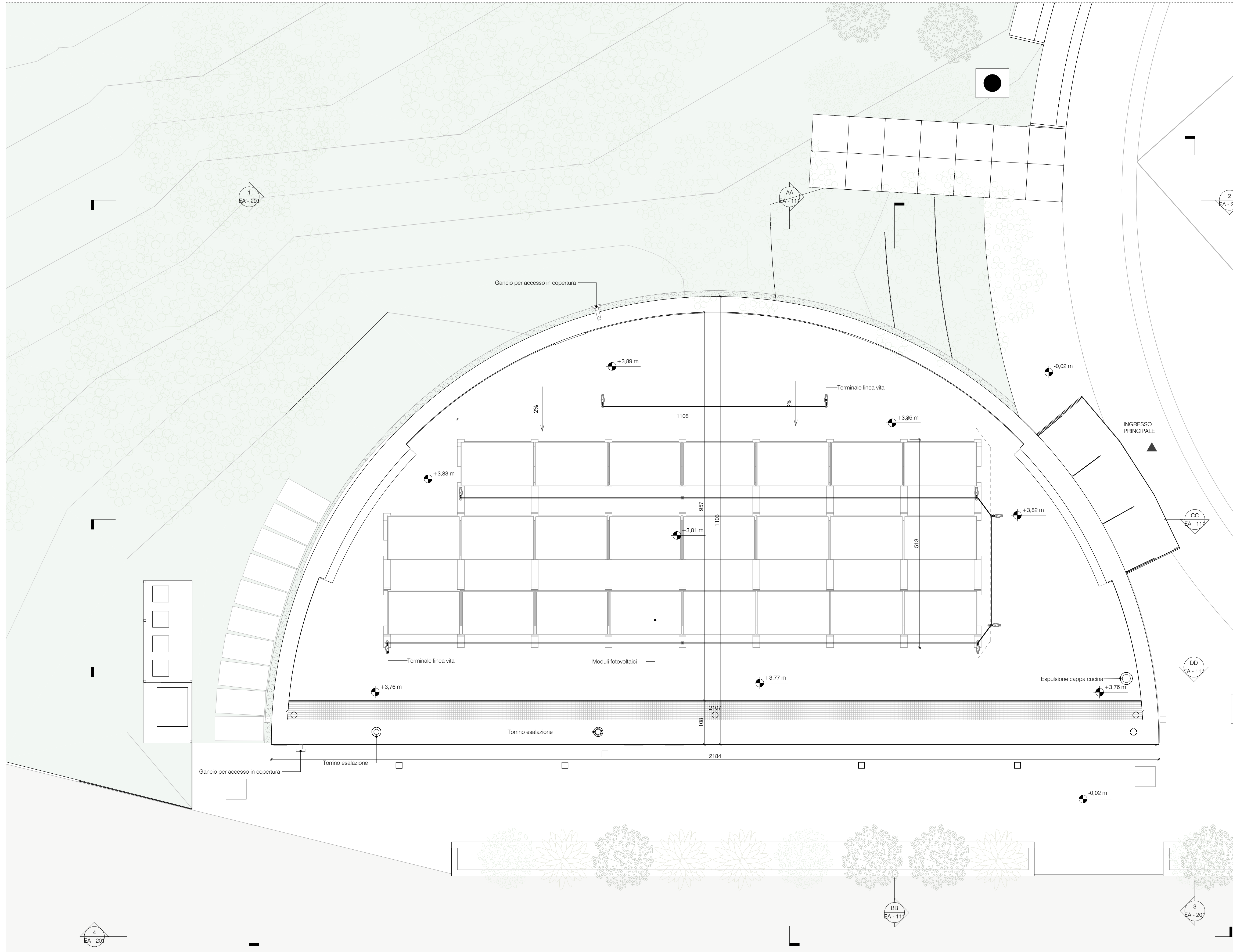
Stato di Progetto - Pianta delle Coperture 1 : 50
