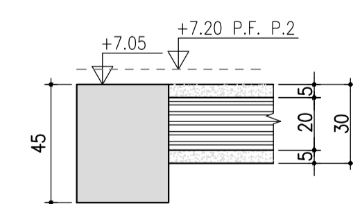
Sez. "F - F" Scala 1:20
