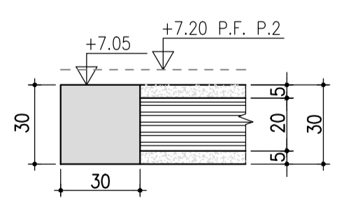
Sez. "C - C" Scala 1:20
