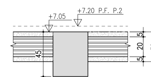
Sez. "G - G" Scala 1:20
