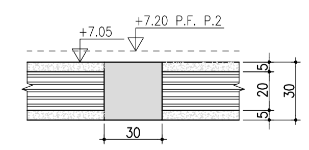
Sez. "D - D" Scala 1:20
