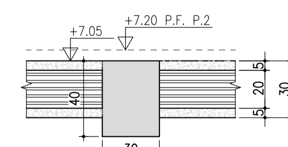
Sez. "E - E" Scala 1:20
