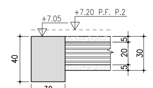
Sez. "H - H" Scala 1:20
